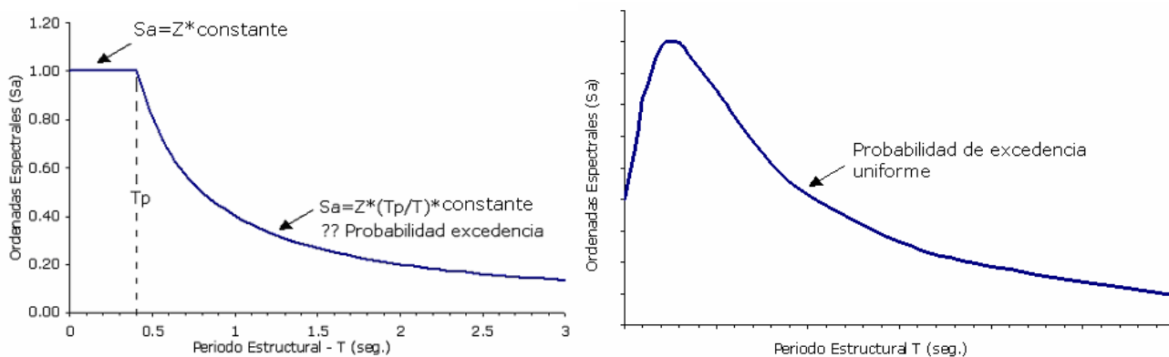
Figura 1.1. Forma espectral obtenida de la norma sísmica Peruana y la que se obtiene del espectro de peligro uniforme.
