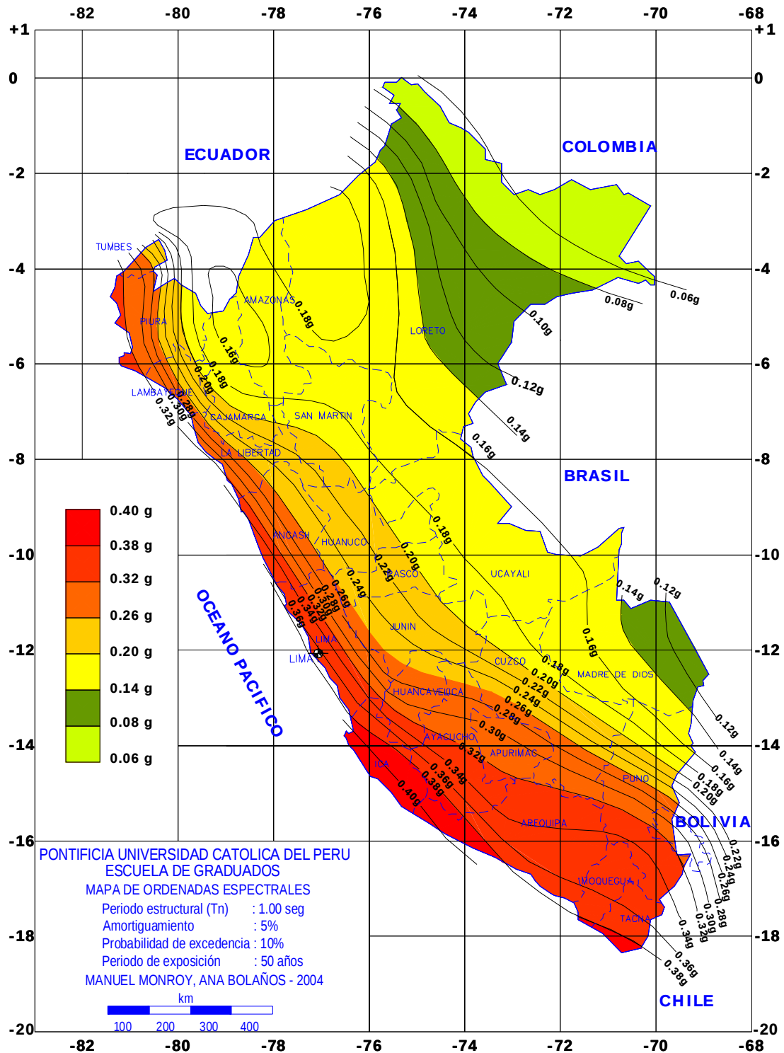
Figura 4.4. Distribución de ordenadas espectrales para el Perú correspondientes a un periodo estructural de 1.0seg con 5% de amortiguamiento y periodo de retorno de 475 años.
