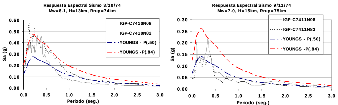
Figura 3.2. Espectros de respuesta registrados en el parque de la Reserva (Lima) vs. el espectro obtenido con el modelo de Youngs para el valor medio P(.50) y el valor medio más la desviación estándar P(.84)
