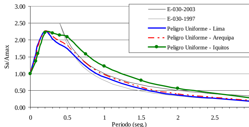
Figura 4.2. Comparación de espectros de diseño propuestos por el código Peruano con los espectros de peligro. Los valores están normalizados a la aceleración máxima del suelo.
