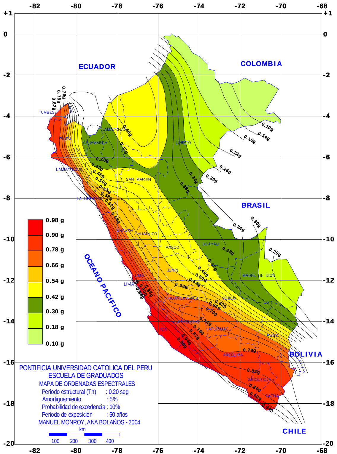
Figura 4.3. Distribución de ordenadas espectrales para el Perú correspondientes a un periodo estructural de 0.2seg con 5% de amortiguamiento y periodo de retorno de 475 años.
