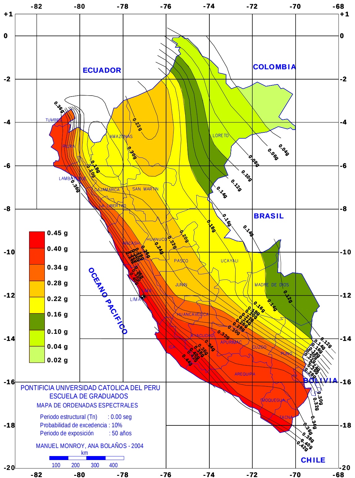
Figura 4.2.- Distribución de ordenadas espectrales para el Perú correspondientes a un periodo estructural de 0.0seg (aceleración del suelo) y periodo de retorno de 475 años.
