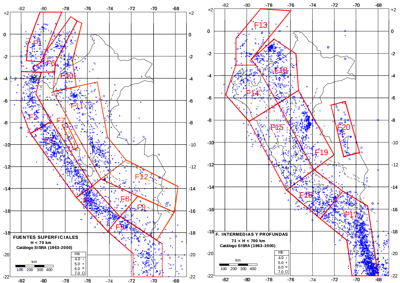
Figura 3.1. Distribución de las fuentes sísmicas de subducción de interfase, intraplaca y fuentes de corteza utilizadas en este trabajo.
