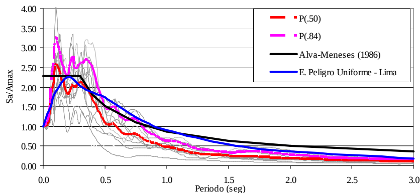
Figura 4.1. Promedio P(.50) y promedio más desviación estándar ( P(.84) ) de los espectros de respuesta de 12 registros sísmicos obtenidos en Lima.
