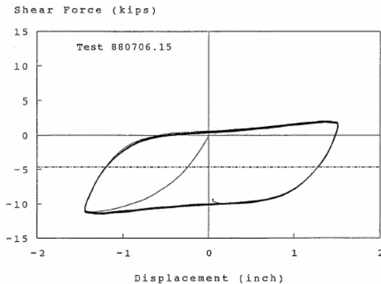
Fig. 3.18. 7-Plate ADAS element hysteretic behavior
