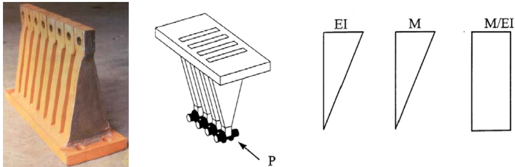
Fig. 3.19. TADAS element
