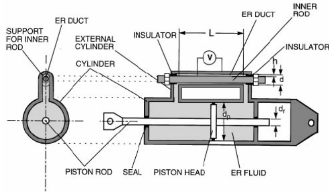
Fig. 6.9. Schematic of the ER Damper
